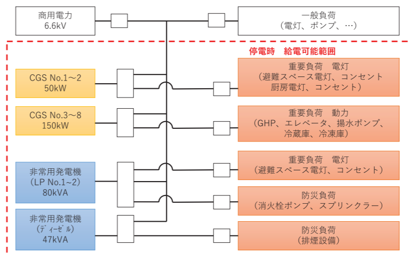
【電気系統図】
