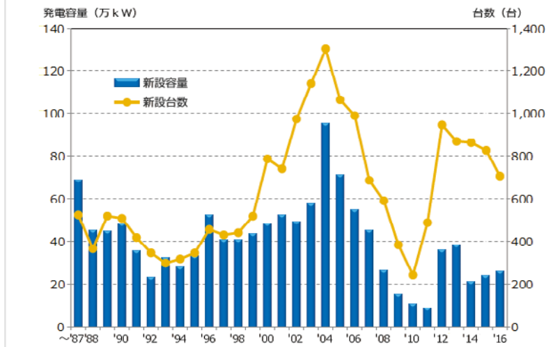
年度別 新規導入容量および台数（撤去含まず）（2017年3月末）
